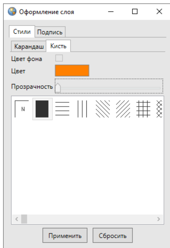
Рис. 2.66: Настройка отображения полигональных объектов. Вкладка «Кисть»
