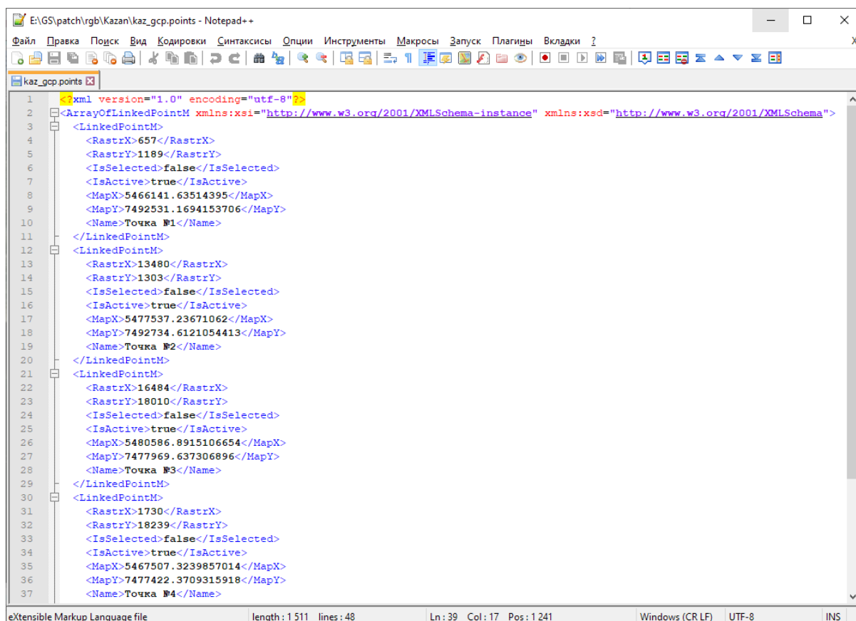
Рис. 2.92: Файл с сохраненными координатами контрольных точек
